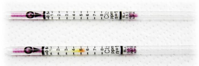
写真：試験結果 (上段：試験前の検知管、下段：試験後の検知管)
